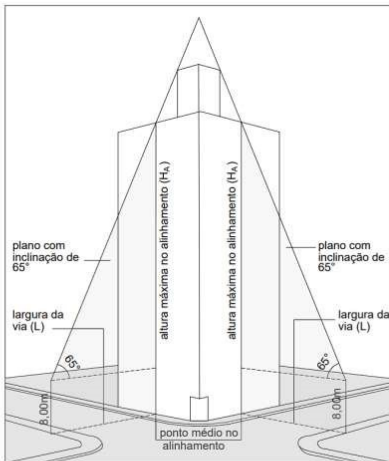
Figura1: Gabarito, altura máxima no alinhamento ( H_A )
