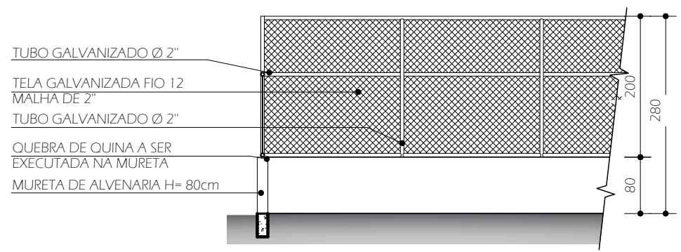
DETALHE ALAMBRADO FUNDOS H=200/280 ESCALA 1:75
