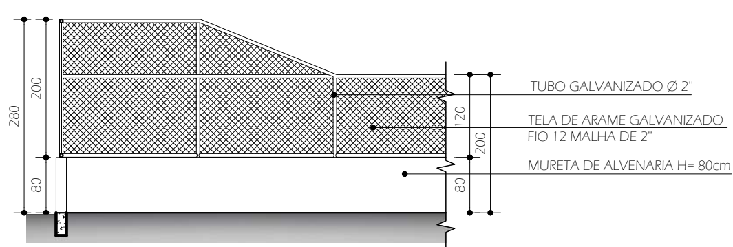
DETALHE ALAMBRADO LATERAL ESCALA 1:75
