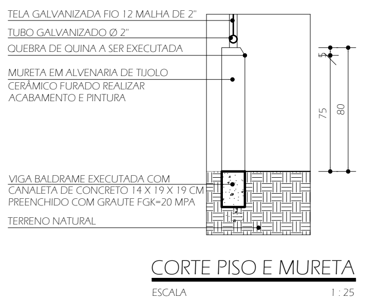
DETALHE PILAR E MURETA ESCALA 1:25
