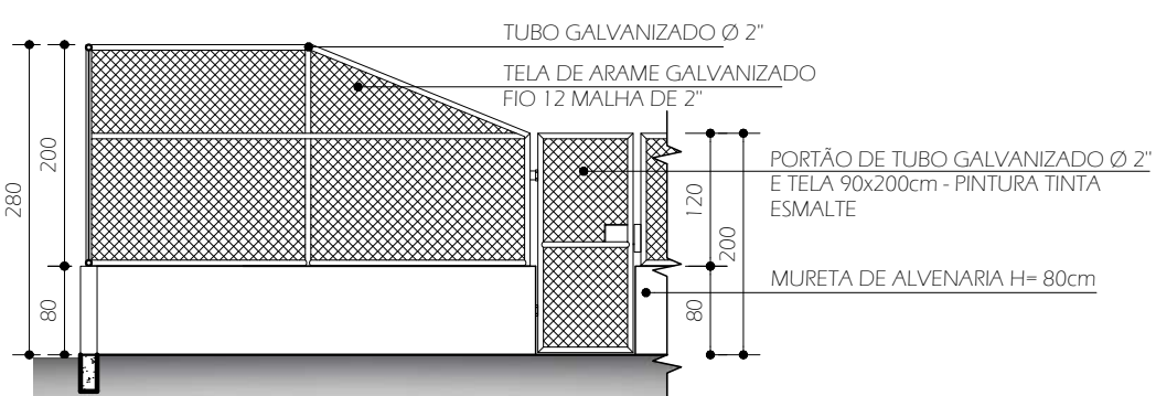
DETALHE PORTÃO E ALAMBRADO H=200 ESCALA 1:75
