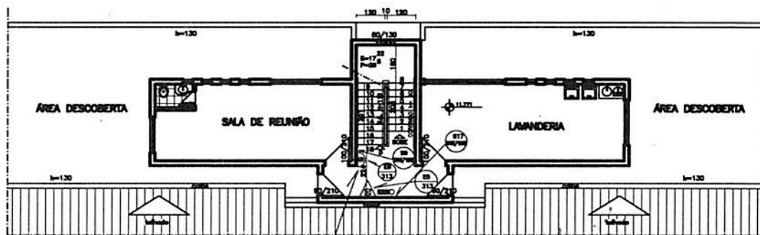
PLANTA 3º PAVIMENTO _ ESCALA 1/100
