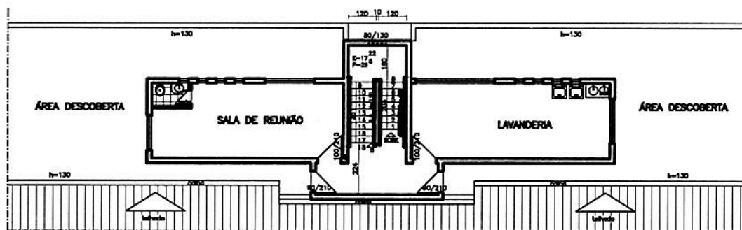
PLANTA 3ª PAVIMENTO _ ESCALA 1/100
