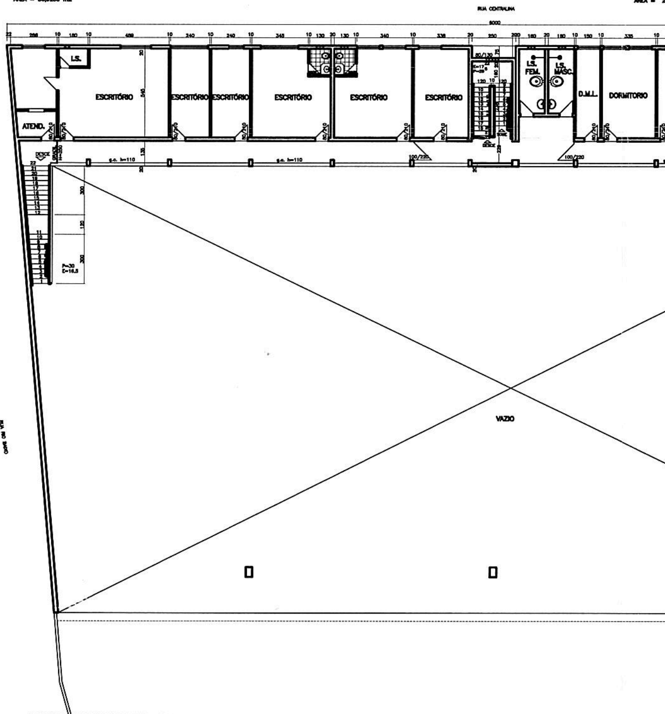
PLANTA 2ª PAVIMENTO _ ESCALA 1/100
